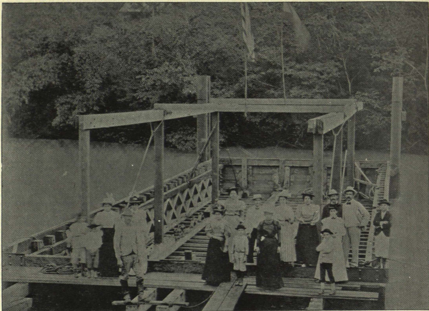
Draga de The Yumary Improvement and Gold Dredging Co. — Fotografía de F. Fajardo Alcáiz, tomada por el frente
